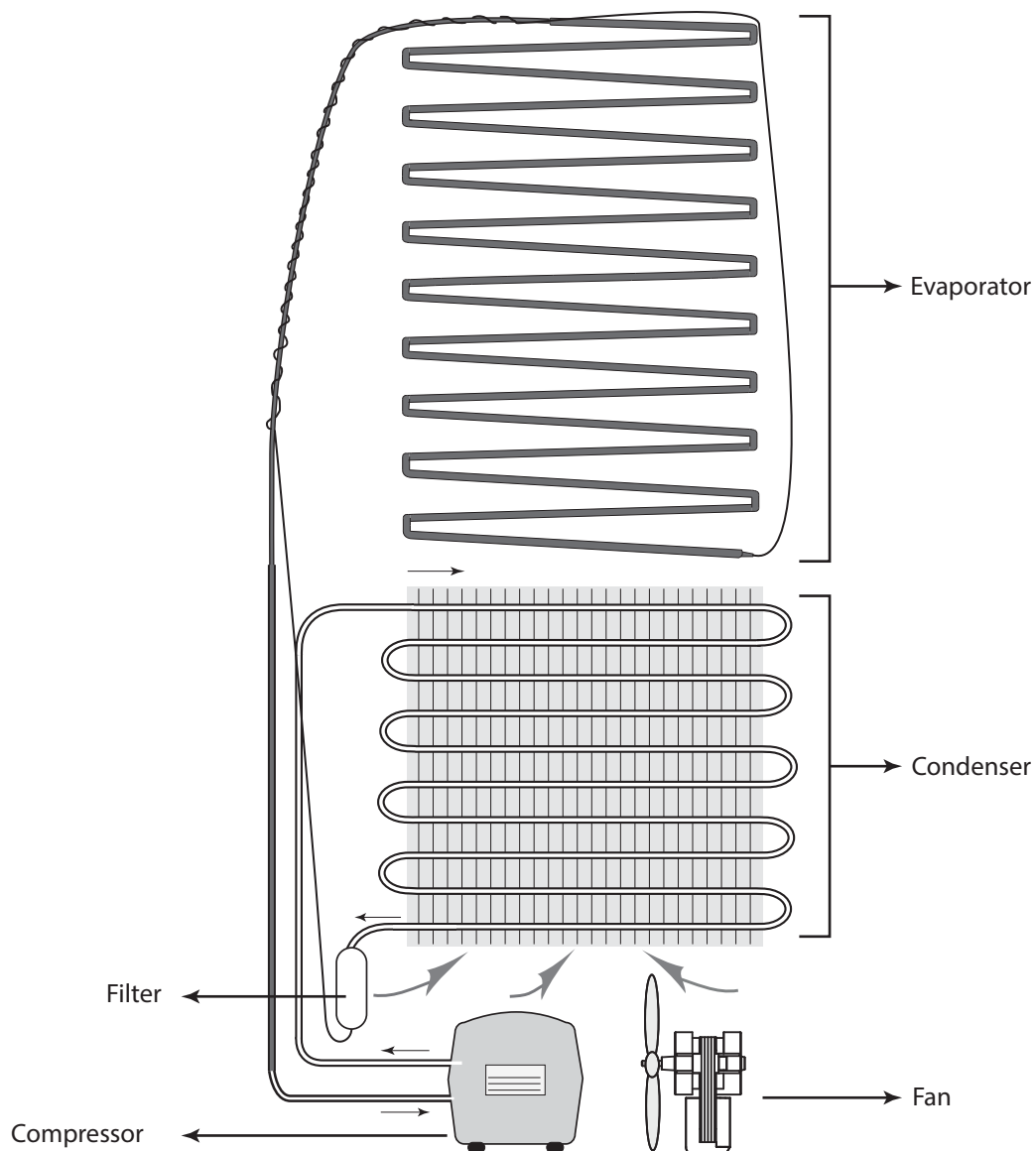
Circuito termodinámico
